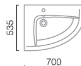
113720 lavatório 70 esquerdo lavabo 70 izquierdo left 70 wash basin lavabo 70 gauche
