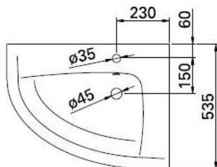
113720 lavatório 70 esquerdo lavabo 70 izquierdo left 70 wash basin lavabo 70 gauche
